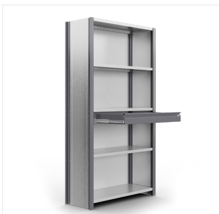
Skuffe Dybde: 400 og 500 mm Bredde: 915 mm
