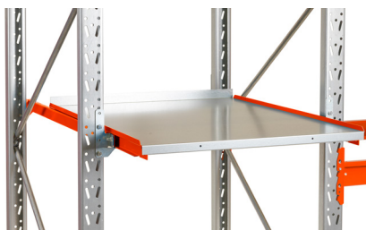
Udtrækshylde for plukgods uden palle
