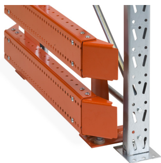
Truckværn højde 400 mm – for ydergavle og truckgennemkørsler. Højde 400 mm
