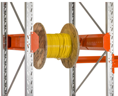
Kabeltromleophæng – med selvlåsende aksel. Justerbar fiksering af kabeltromle samt flytbar akselplacering i dybden. For sektion 950 mm og 1350 mm.
