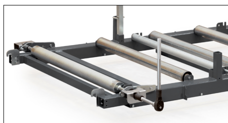
Drivpakke på lastbæreren som letter indlastningen
