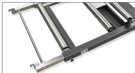
Kroge i forkant af lastbærer
